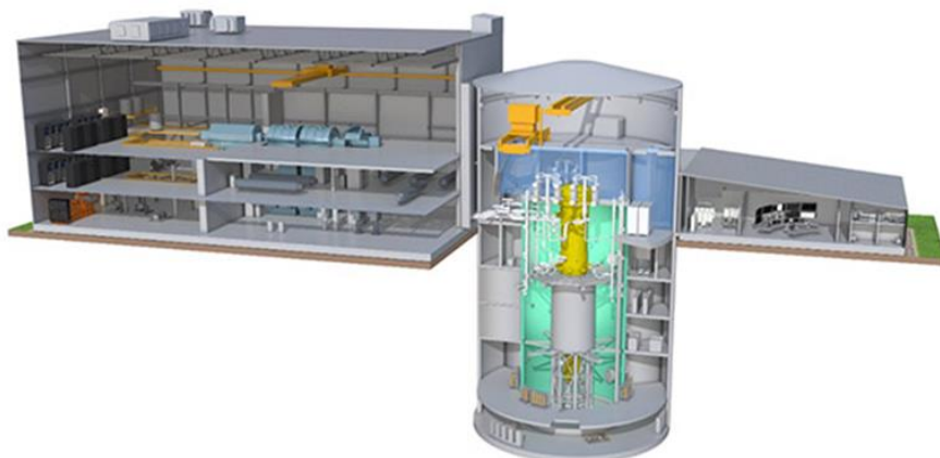
Figuur 2 Doorsnede BWRX
